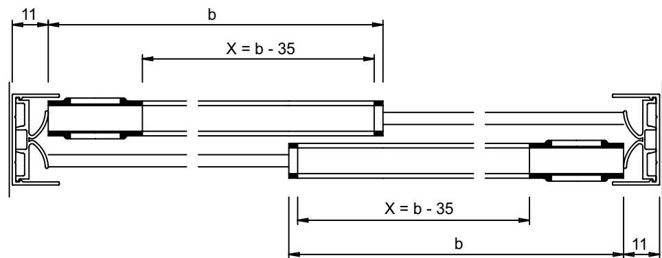
loopprofiel met zamak slotbehuizing en slot adapter
