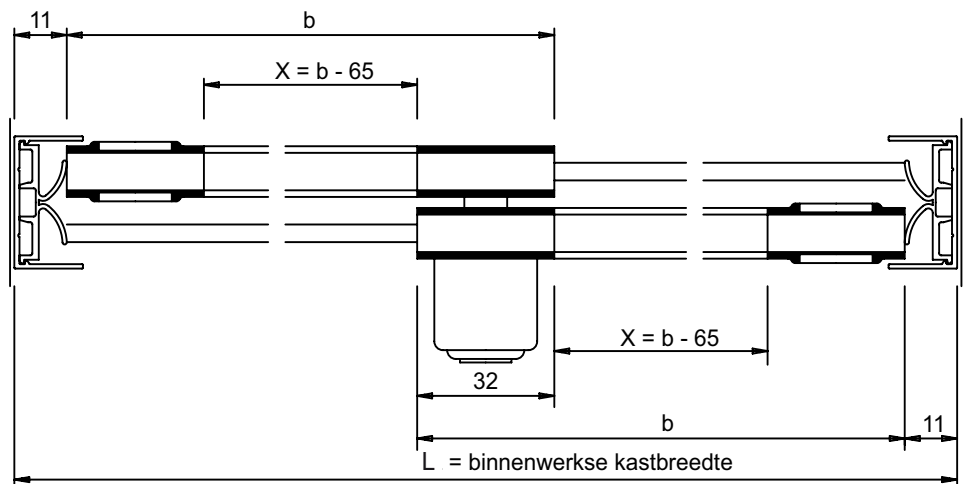
loopprofiel met zamak slotbehuizing en slot adapter
